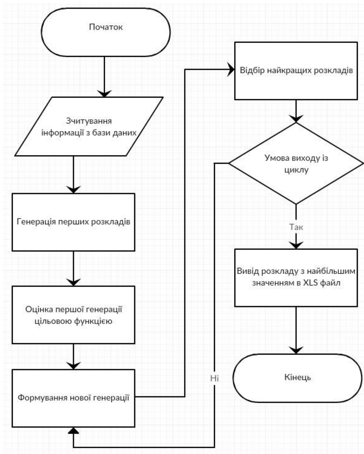
Рисунок 2.3 – Блок-схема алгоритму формування розкладу
