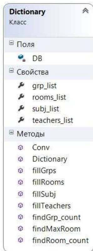
Рисунок 3.3 – Клас Dictionary
