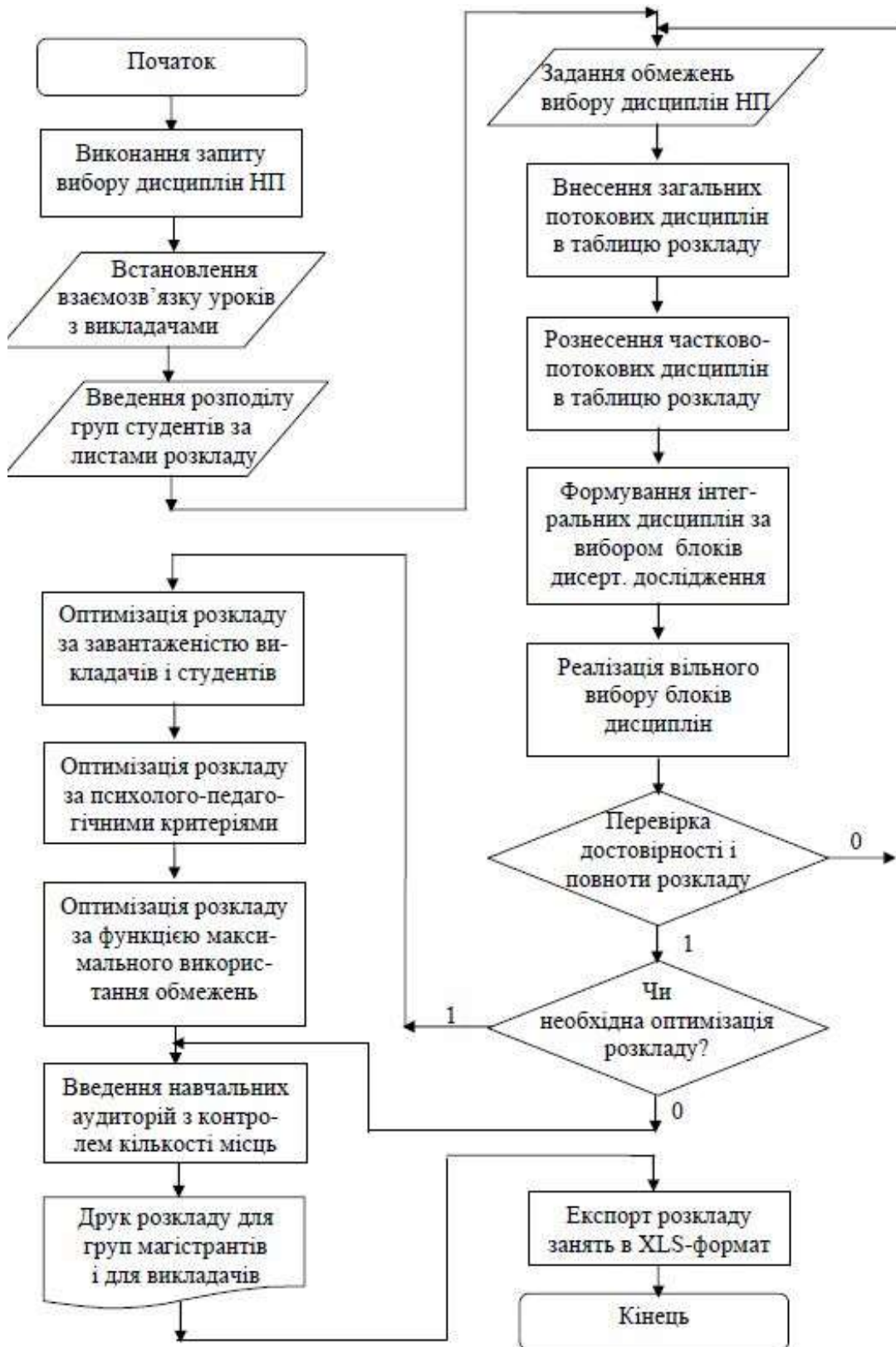
Рисунок 1.1 - Алгоритм реалізації методу формування розкладу магістратури. [3]
